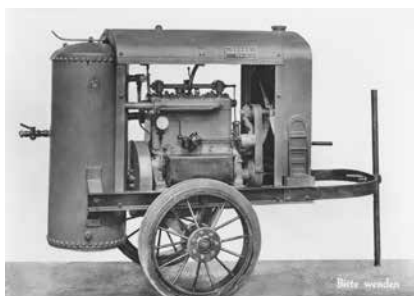
Compresseur RUBAG Zurich, 1930
